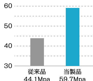
ヨコ方向の引っ張り強さ
